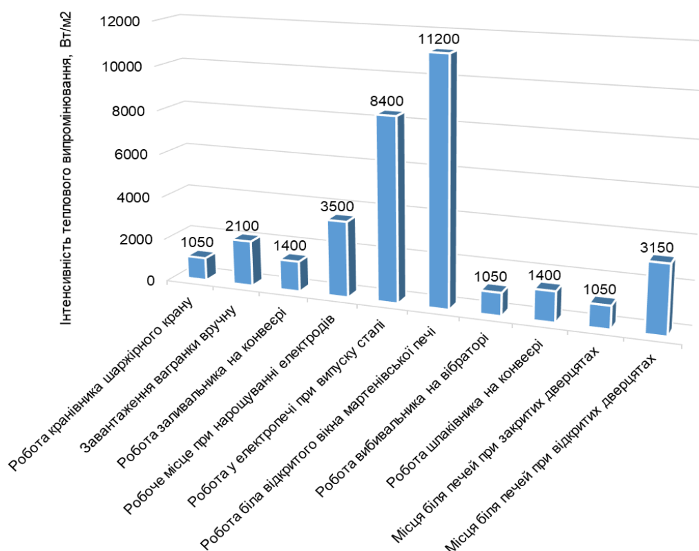
Рис. 1 – Інтенсивність теплового потоку на робочих місцях в ливарних цехах.
