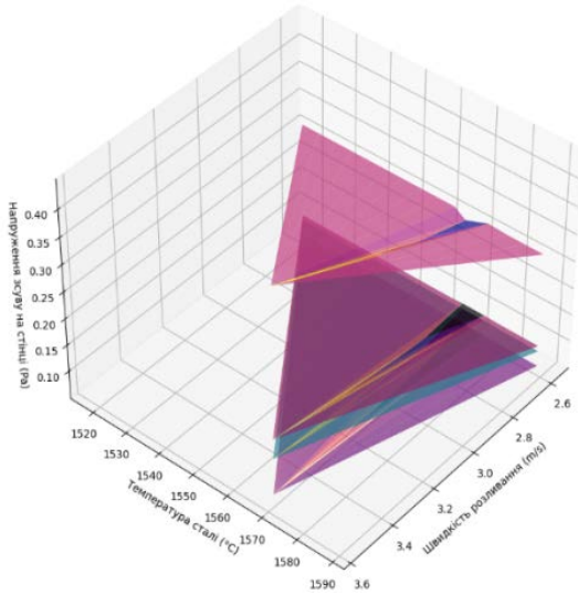
Залежність Напруження зсуву від температури та швидкості розливання (Зони 1-4)
