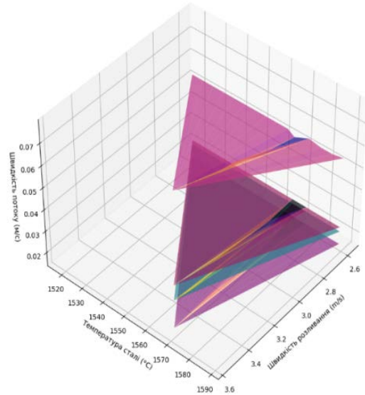
Залежність Швидкості потоку від температури та швидкості розливання (Зони 1-4)
