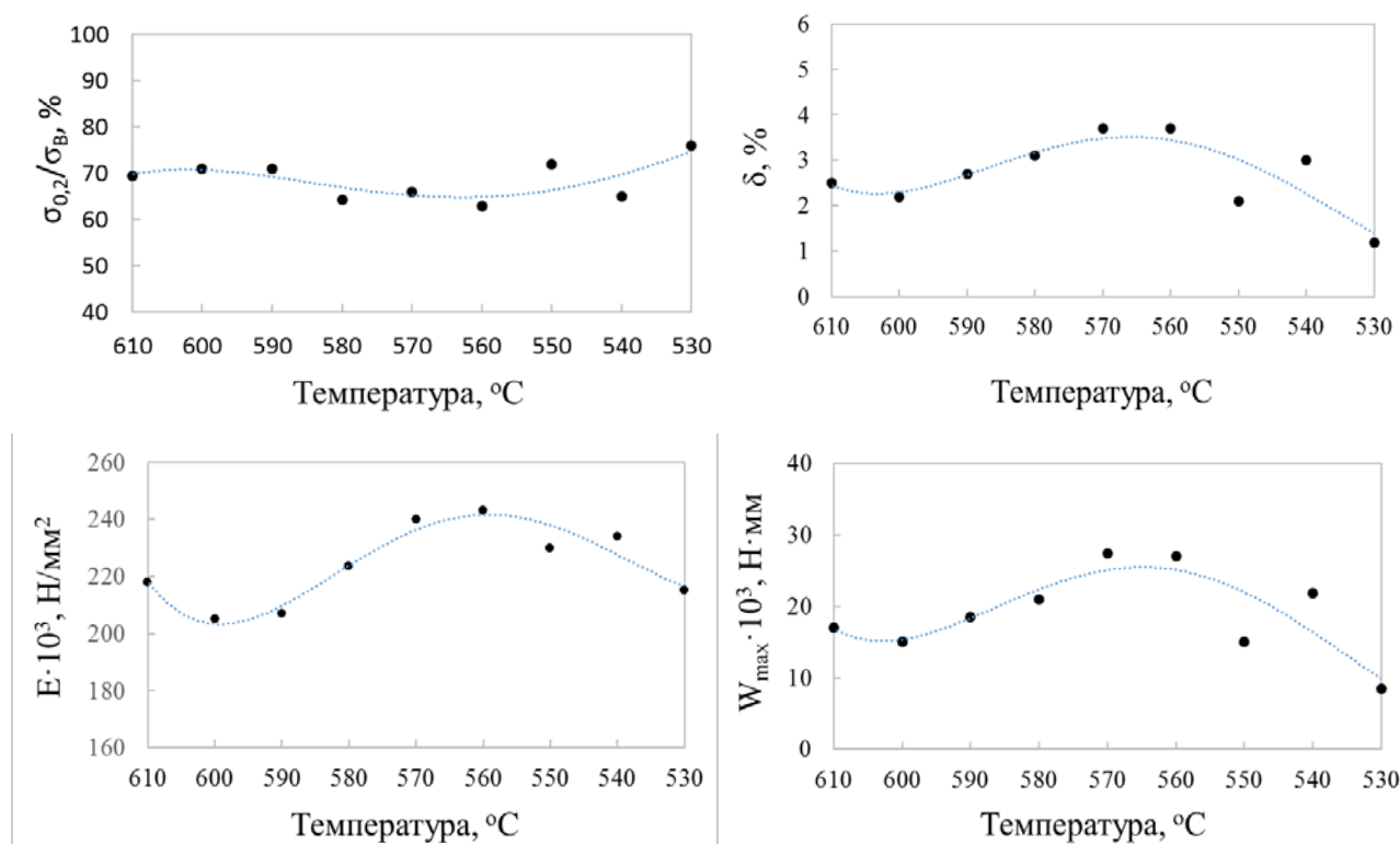
Рисунок 1 – Залежність механічних властивостей сталі C80D2 від температури патентування
