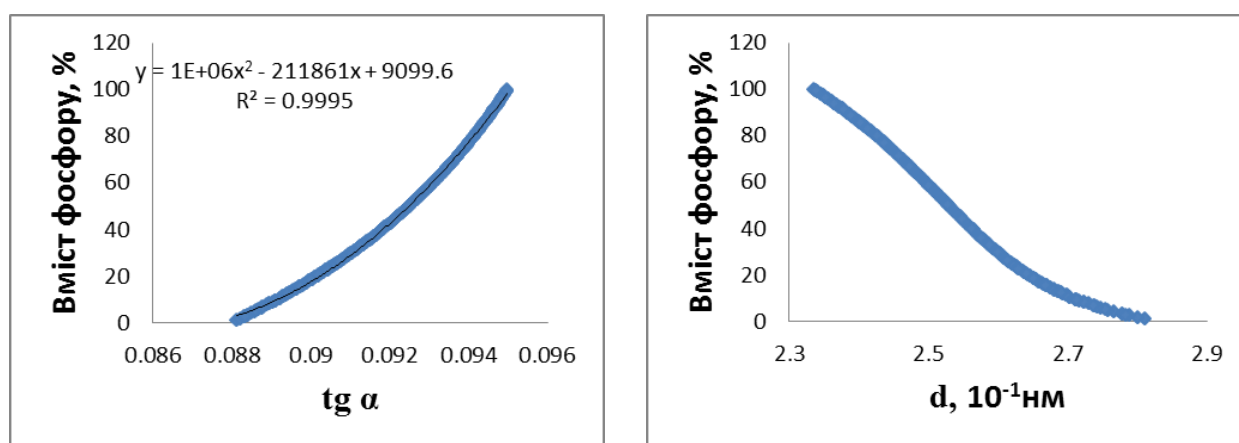
Рисунок 2 – Взаємозв'язок між зміною вмісту фосфору в системі Fe-P та параметрами міжатомної взаємодії ( \text{tg}\alpha і d )
