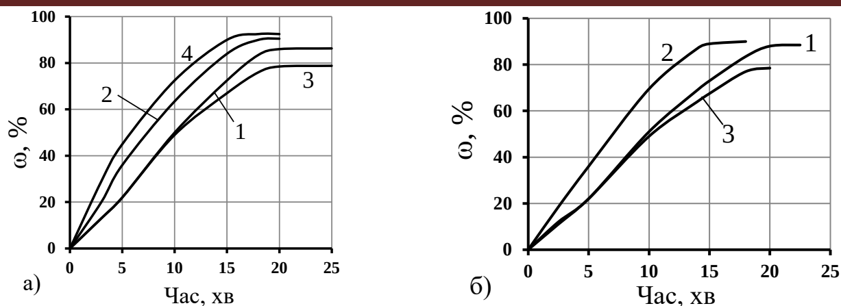
Рисунок 2. Вплив хлоридів лужних металів на кінетику окислення заліза при температурах, що відповідають при T_{ок} (а) і при 623 К (б); залізо отримано відновленням Fe_2O_3 монооксидом вуглецю при 1073 К: 1 – без добавки, 2 – 1 % KCl, 3 – 1 % LiCl, 4 – 3 % KCl
