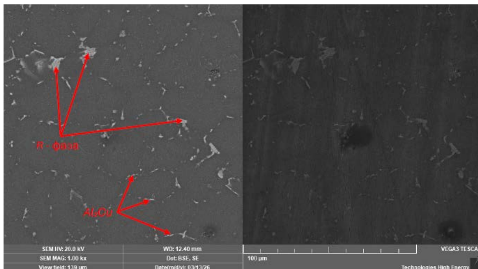
Рис. 1 – Електронно-мікроскопічне зображення мікроструктури сплаву Al – 5 % Cu – 0,8 % Mn – 0,25 % Ti
