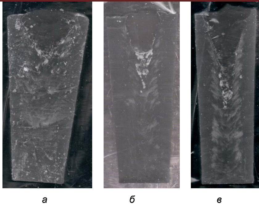
Рисунок 2 – Зразки кута сходження у усадкової раковини
