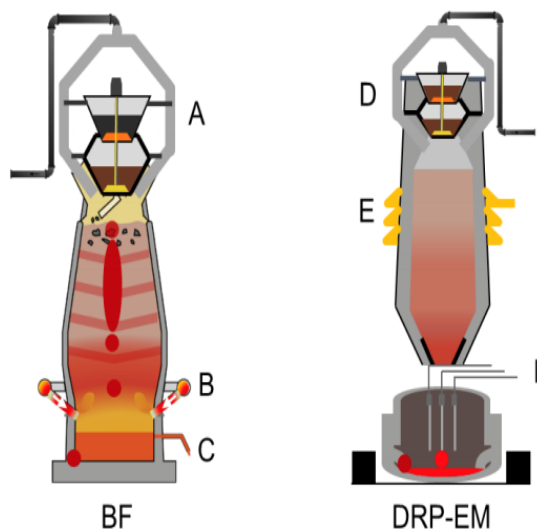
Рисунок 1 – Варіанти отримання заліза процесами BF та DRP-EM
