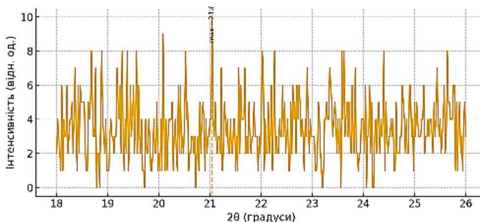
Рис. 2 – Дифрактограма сплаву 4 в області 18 – 26 град
