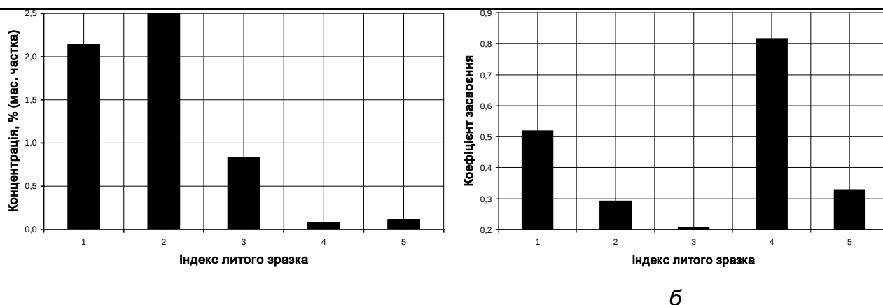
Рис. 1. Показники засвоєння елементів матричним розплавом із дисперсно-наповненої газмоделі [1]: а – концентрації елементів-модифікаторів і легувальних елементів, б – коефіцієнти засвоєння легувальних елементів та елементів-модифікаторів; 1 – кремнію, 2 – міді, 3 – хрому, 4 – ванадію, 5 – титану
