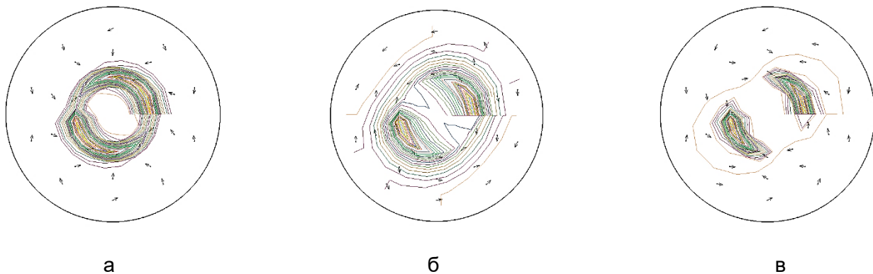
Рисунок 1 – Результати математичного моделювання з відображенням напрямку та розкриття газових потоків при обертанні фурми з Т-подібним наконечником у різних перетинах за висотою ковшу
