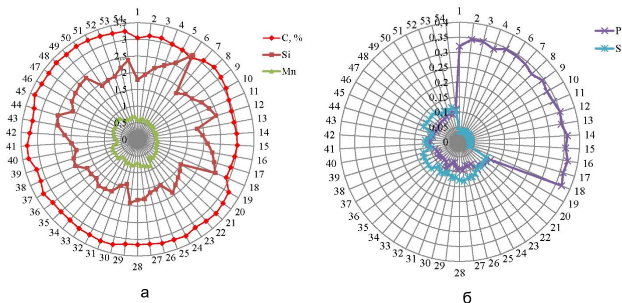
Рис. 1 – Діаграми хімічного складу чавуну ваграночної плавки:
