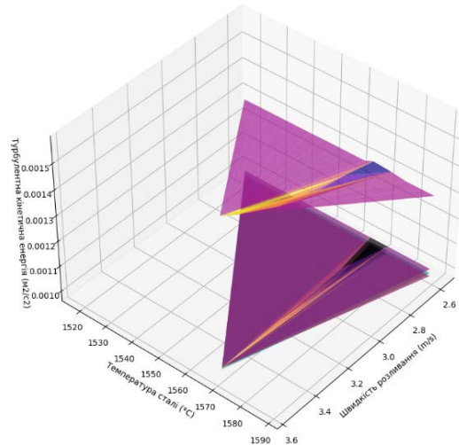
Рисунок 7 Залежність турбулентної кінетичної енергії від температури та швидкості розливання
