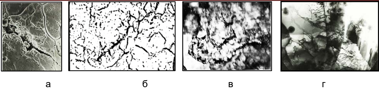
Рис.1 - Тріщини (а) та утворення вторинних зеренних границь у відцентроволитому виливку (б – г); а – х500, б, в - х2000, г - х 20000.
