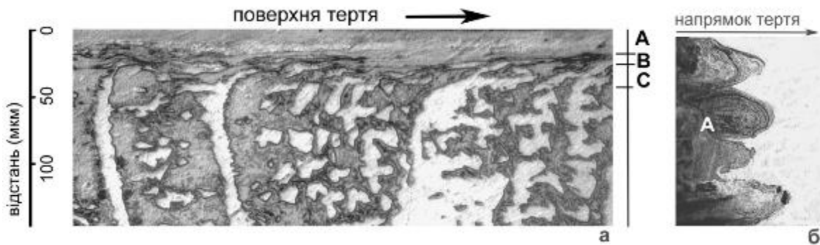
Рис. 3 – Мікроструктура контактної зони литої бронзи в парі тертя Ст45 – лита бронза при вмісті олова 20 ваг %. Швидкість ковзання 4 м/с, навантаження 150 Н. Торцевий шліф а), та косий шліф поверхні тертя пари Ст45- лита бронза, x400 б).
