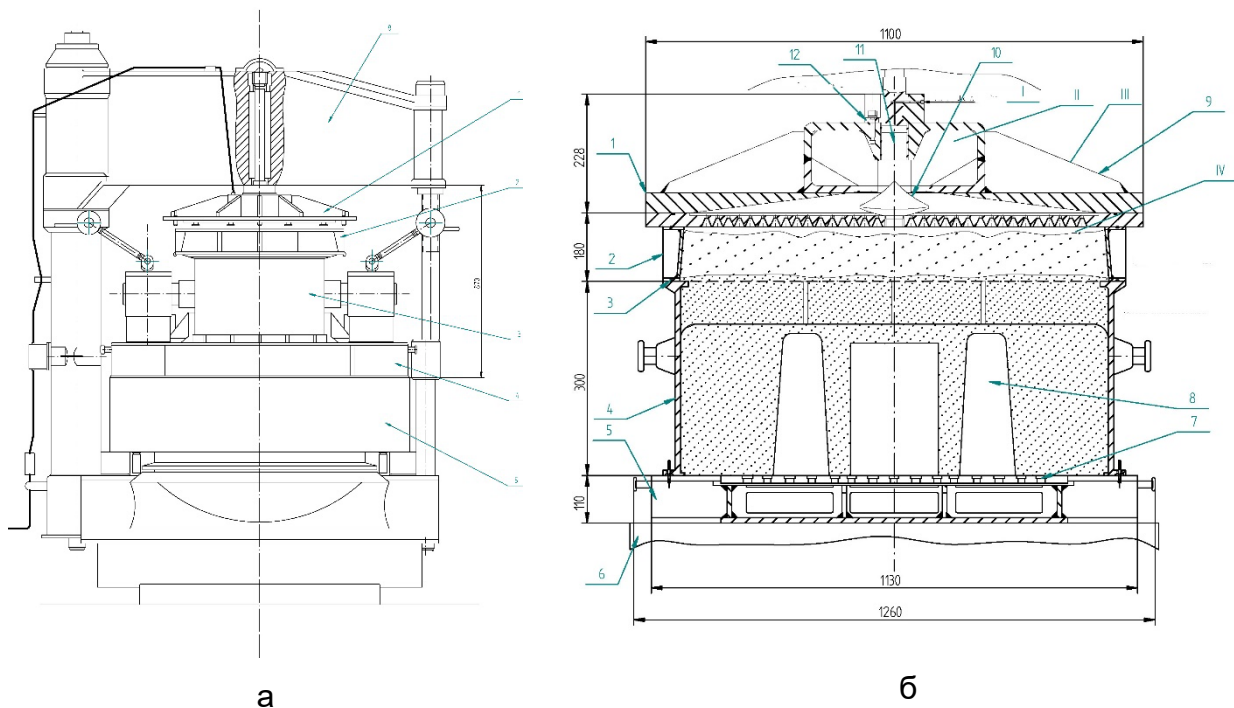
Рис. 1 – Конструкційні рішення по імпульсній машині: а – конструкція машини: 1 – імпульсна камера, 2 – рамка наповнювальна, 3 – опока, 4 – плита підмодельна, 5 – стіл, 6 – затискувач ексцентриковий, 7 – затискувач рамки наповнювальної, 8 – траверса; б – імпульсна камера: 1 – головка пневматична, 2 – рамка наповнювальна,
