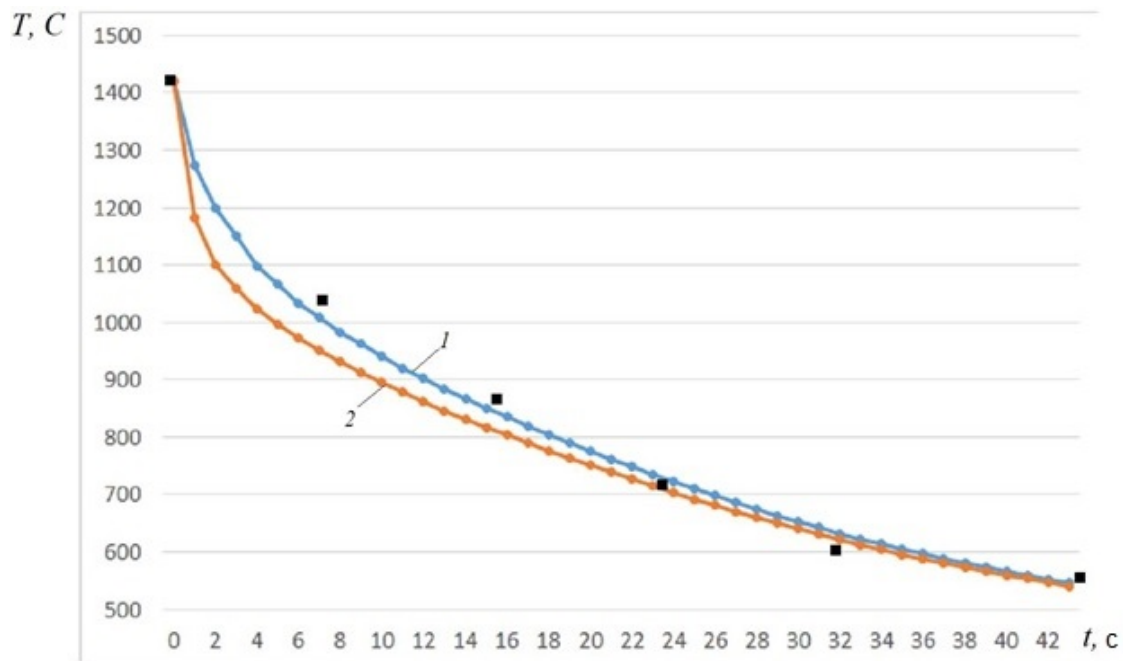
Рис. 1 – Розрахункова зміна температури поверхневого шару виливка кулі Ø40 мм та зазору з газом і кокільною фарбою (чавун виробу: 2,5 % C, 1 % Si; товщина стінки сферичної моделі чавунного кокіля – 40 мм)
