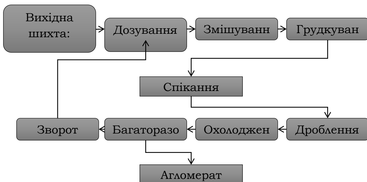
Рисунок 1 – Технологічна схема виробництва агломерату
