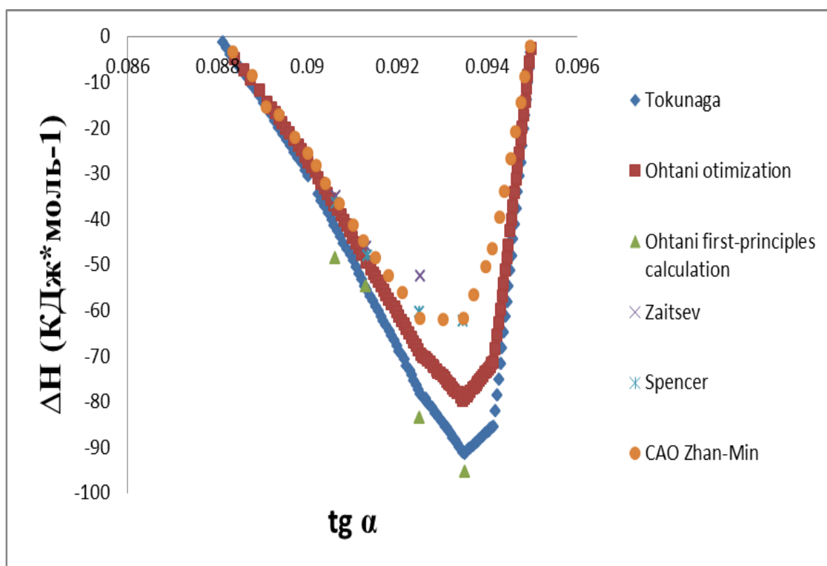
Рисунок 1 – Залежність ентальпії ( \Delta H ) утворення фаз в системі Fe-P від її хімічного складу, представленого параметром міжатомної взаємодії \text{tg } \alpha при температурі 298 K
