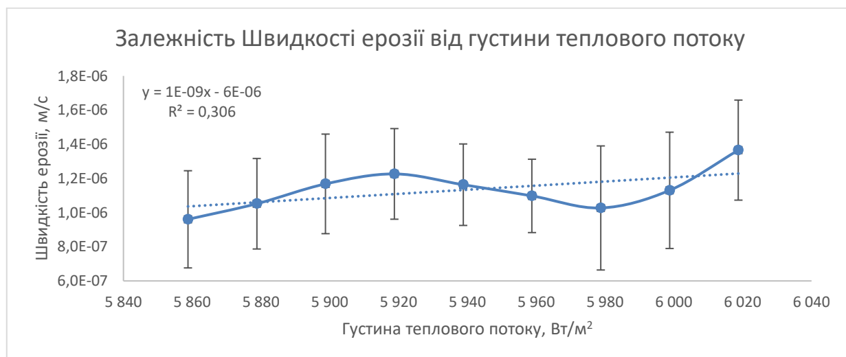
Рисунок 3 – Залежність швидкості ерозії від густини теплового потоку
