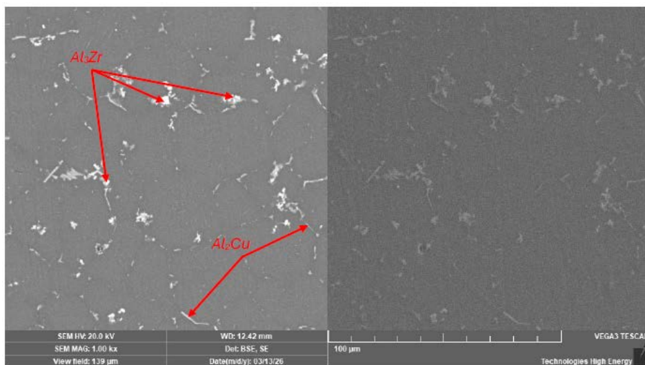
Рис. 3 – Електронно-мікроскопічне зображення мікроструктури
