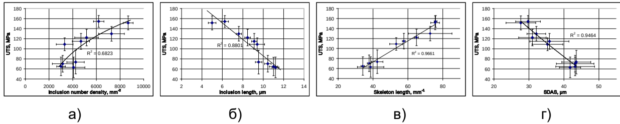
Рис. 2. – Зв'язок \sigma_B із мікроструктурними характеристиками: а) щільність включень; б) довжина включень; в) довжина дендритного скелету; г) відстань між гілками дендритів другого порядку
