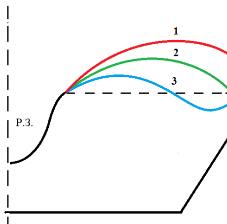
Рисунок 1 – Характеристики хвиль, що утворюються при продуванні рідкої ванни
