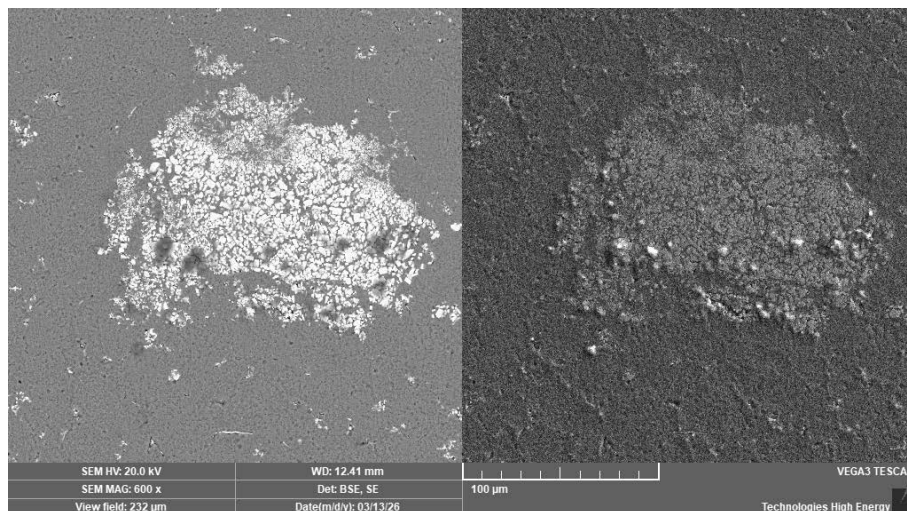
Рис. 4 – Електронно-мікроскопічне зображення мікроструктури сплаву Al – 5 % Cu – 0,8 % Mn – 0,25 % Ti зміцненого цирконієм із ZrF 4 (2,5 %) у зоні надмірно збагаченій цирконієм.
