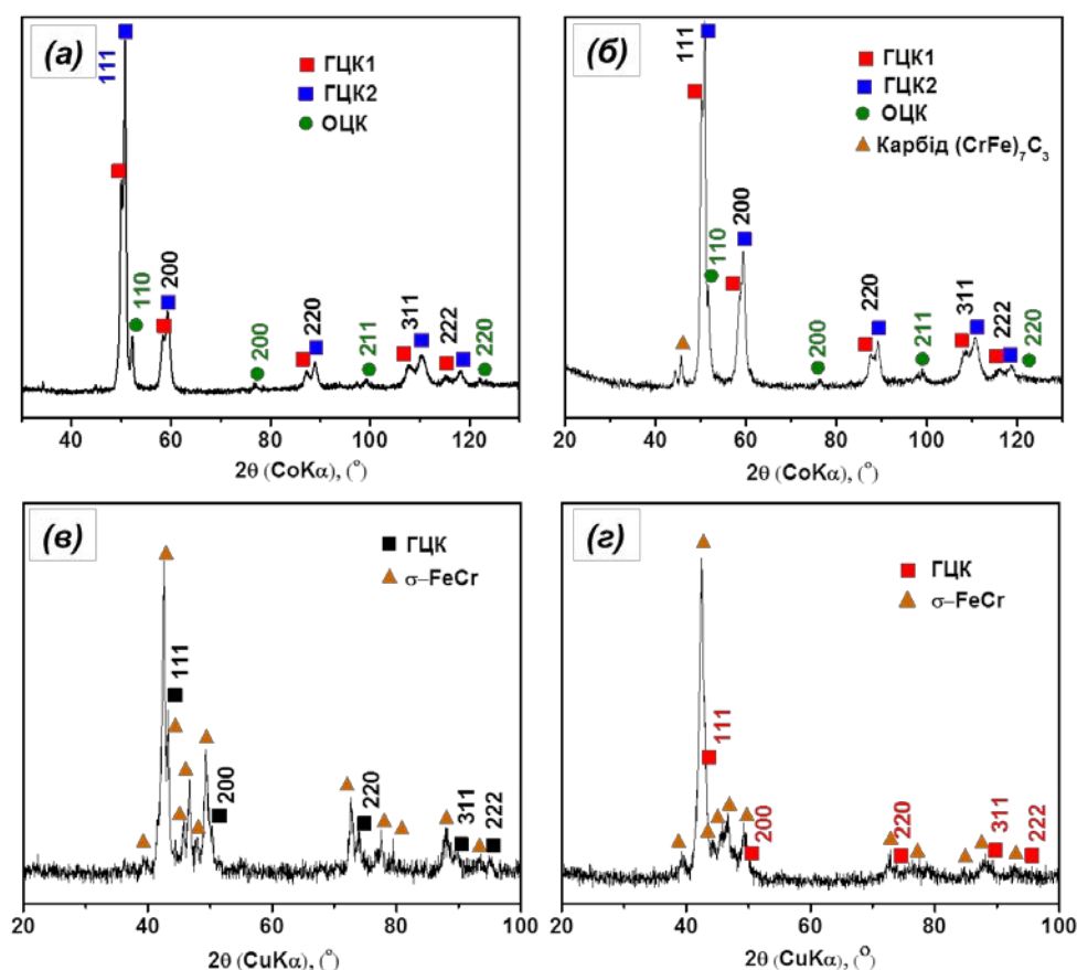
Рис. 1 – Дифрактограми високоентропійних сплавів системи \text{FeNiCrCuMnV}_x (x %, відн. ат. част.): плавка на повітрі а – x= 2,5, б – x= 5, в – x= 10, г – x= 15.
