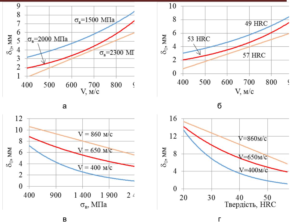
Рис. 1. Вплив швидкості кулі (а, б), межі міцності на розтяг (в) і твердості (г) сталі на балістичну стійкість сталевих пластин.
