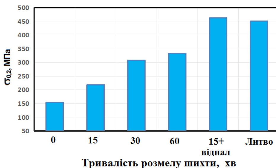
Рис. 1. Залежність границі плинності сплаву при температурі 1000 °С від режимів обробки вихідної шихти
