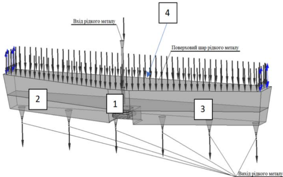
Рисунок 1 – Зонування проміжного ковша за подібністю гідродинамічних показників
