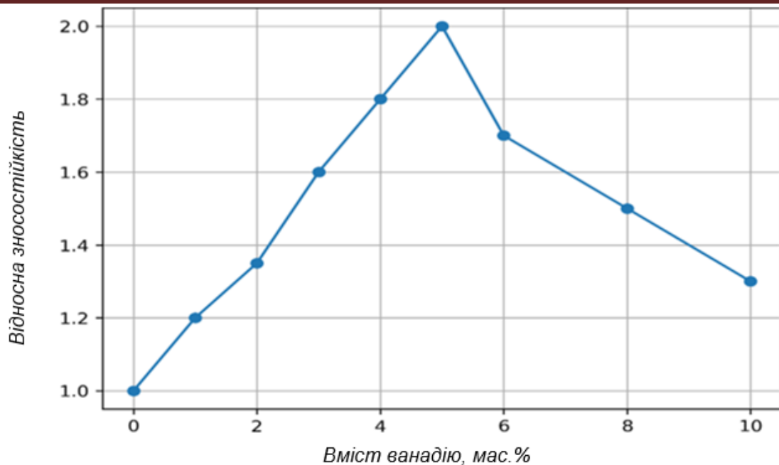
Рис. 1 – Вплив вмісту ванадію на ударно-абразивну зносостійкість хромистих чавунів (узагальнені експериментальні дані) [1].
