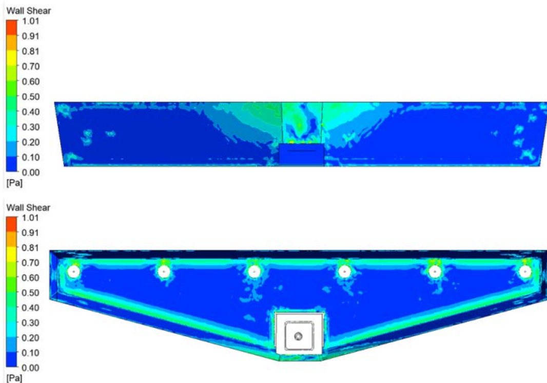
Рисунок 1 – Розраховане напруження зсуву зони дельти і випускних отворів проміжного ковша
