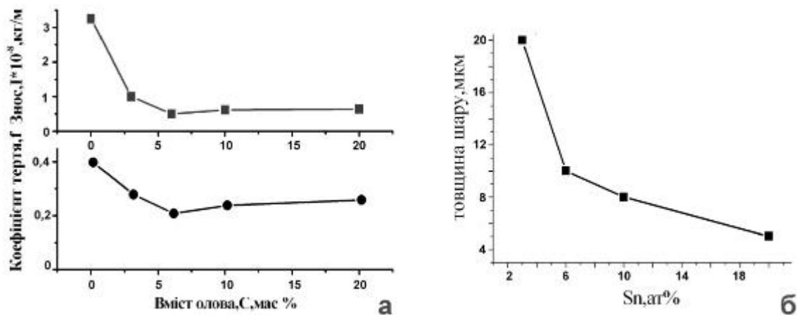
Рис. 2 – Залежність зносу та коефіцієнта тертя при терті пари Ст45- лита бронза від вмісту олова (а), та товщина шару тертя на литій бронзі в парі тертя Ст45 - лита бронза з вмістом 3 ваг% Sn, 6 ваг% Sn, 10 ваг% Sn та 20 ваг% Sn), швидкість ковзання 4м/с. Навантаження 150 Н (б).
