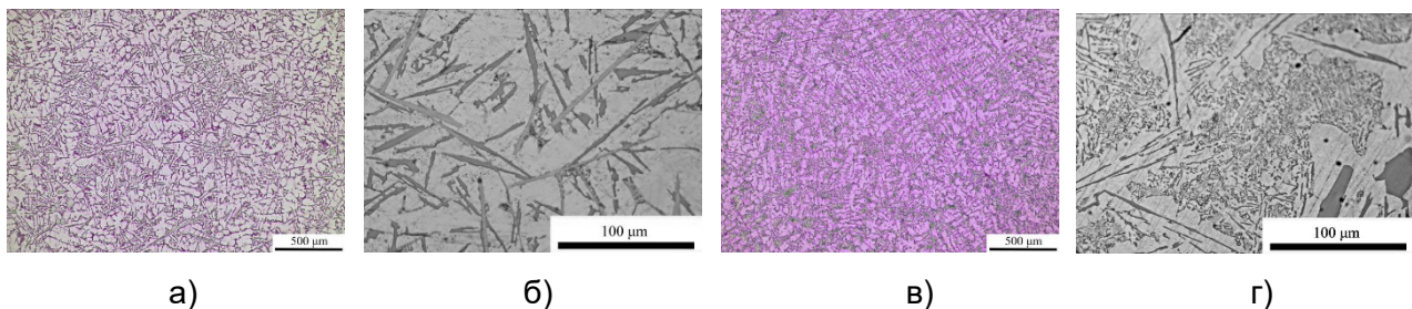
Рис. 1. – Вплив вібраційної обробки розплаву на мікроструктуру силуміну: а, б) без обробки, збільшення \times 50 (а) та \times 500 (б); в, г) вібрація 180 Гц, зі скважністю 50 %, збільшення \times 50 (в) та \times 500 (г).
