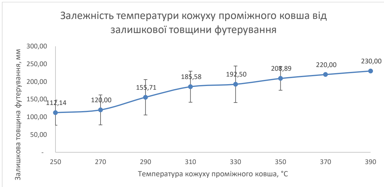
Рисунок 1 – Залежність товщини зношеного шару футерування впродовж серії розливання від температури кожуху проміжного ковша
