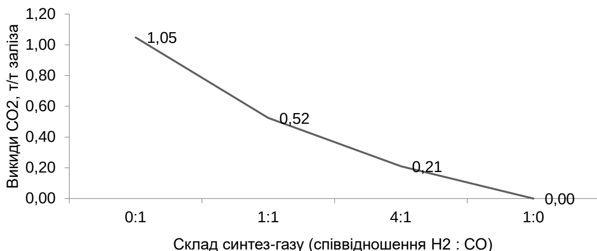
Рис.1 – Залежність викидів парникового газу від складу синтез-газу в процесі прямого відновлення заліза
