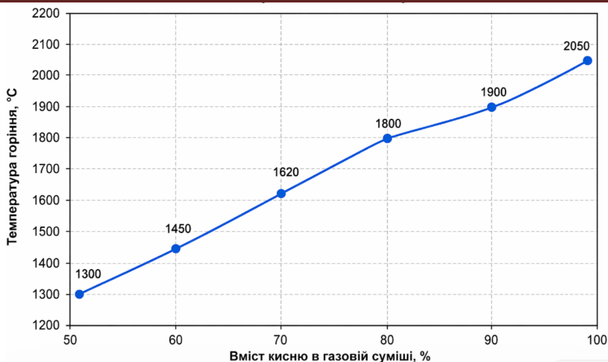
Рисунок 1 – Залежність температури горіння CO від вмісту кисню в газовій суміші (графік: вісь X – вміст O_2 , %, вісь Y – температура, °C; крива зростаюча)
