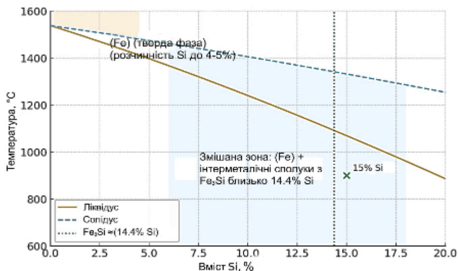
Рис. 1. Вплив вмісту Si у Fe–Si сплаві на температуру ліквідусу та утворення інтерметалідних фаз [9]
