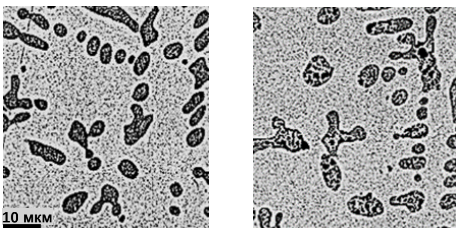
Рис. 2 - Особливості структури вкраплень заліза в сплаві системи Cu-Fe, отриманого в ливарних формах: а) без дії постійного магнітного поля; б) під дією постійного магнітного поля.
