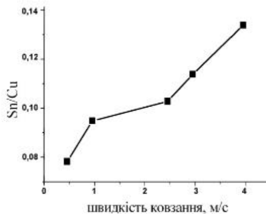
Рис. 4 – Співвідношення атомів олова та міді в шарах тертя на литій бронзі в парі тертя Ст-45- лита бронза (з вмістом 3 ваг% Sn, 6 ваг% Sn, 10 ваг% Sn та 20 ваг% Sn) в залежності від швидкості ковзання. Навантаження 100 Н.
