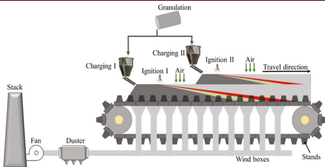
Рис. 1 – Схема процесу двошарового спікання
