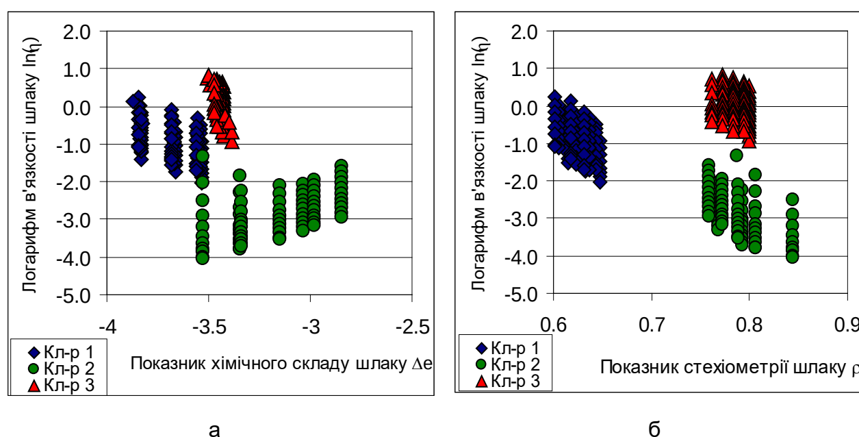
Рисунок 2 – Зв'язок в'язкості з інтегральними показниками складу шлаку по результатам кластеризації масиву даних фосфоровмісних шлаків
