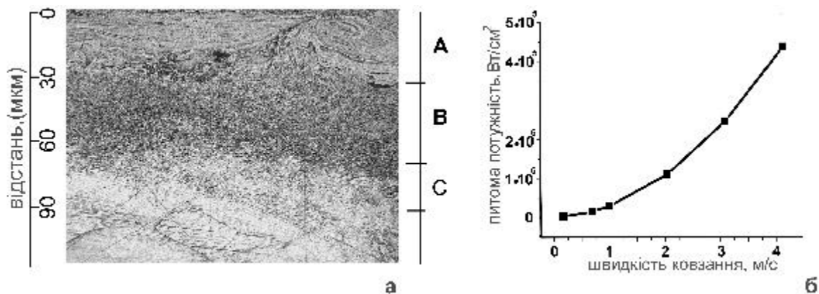
Рис. 1 – Мікроструктура поверхні литої міді в парі тертя Ст.45 - лита мідь, торцевий зріз, швидкість ковзання 3 м/с, навантаження 100 Н (а), та залежність питомої потужності удару двох мікро виступів у момент зіткнення від швидкості ковзання для пари тертя Ст.45 – лита мідь (б).
