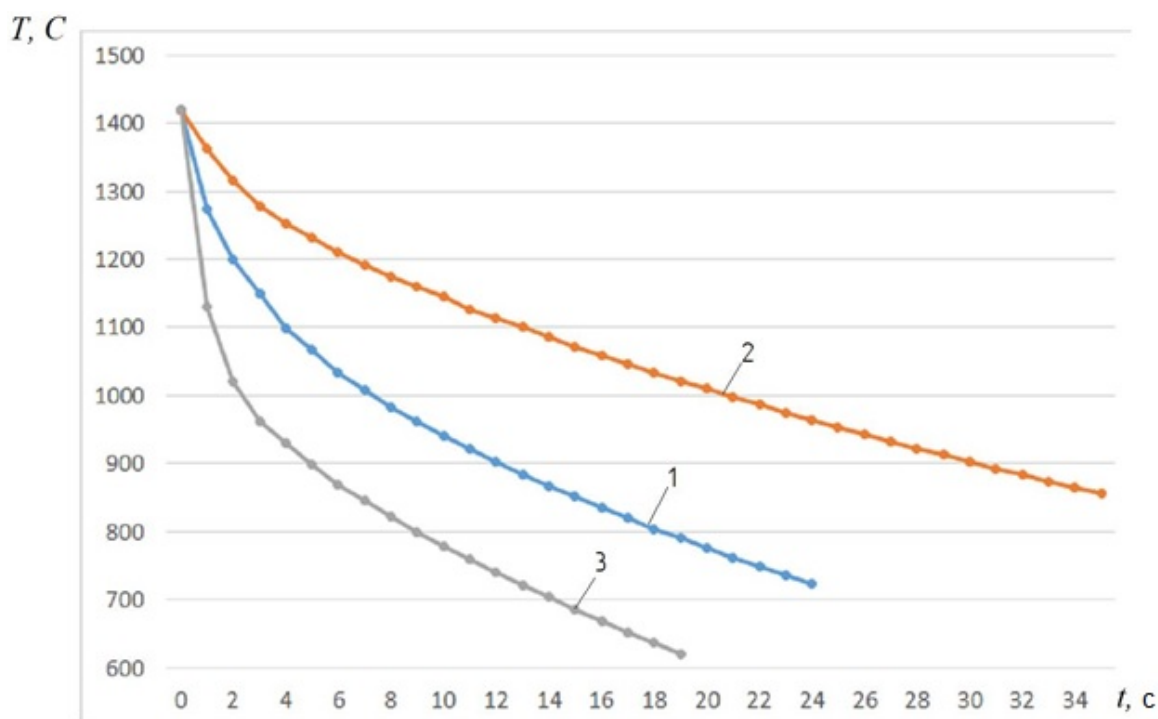
Рис. 2 – Розрахункова зміна температури поверхневого шару виливка кулі \varnothing 40 мм до повного затвердіння (чавун виробу: 2,5 % C, 1 % Si; товщина стінки сферичної моделі чавунного кокіля – 40 мм)
