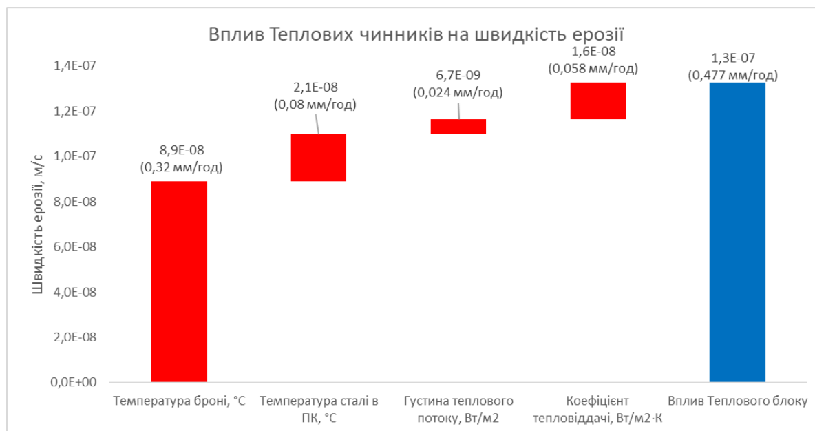
Рисунок 1 – Відносний аналіз важливості теплових факторів моделі на швидкість ерозії проміжного ковша.
