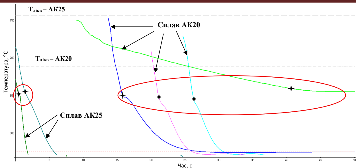
Рис.2 - Криві охолодження алюмінієвих сплавів АК20 та АК25 отримані в різних умовах охолодження
