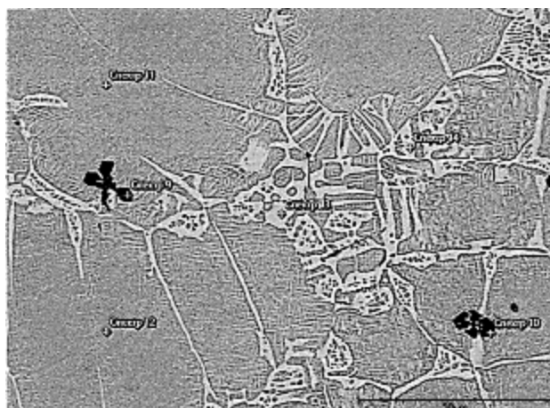
Рис. 3 – Мікроструктура сплаву 4
