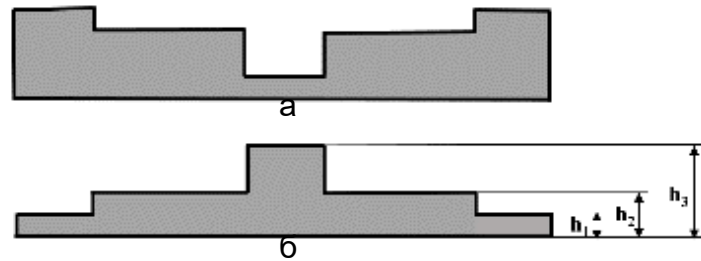
Рис. 1 - Переріз форми (а) і експериментального зразка (б).
