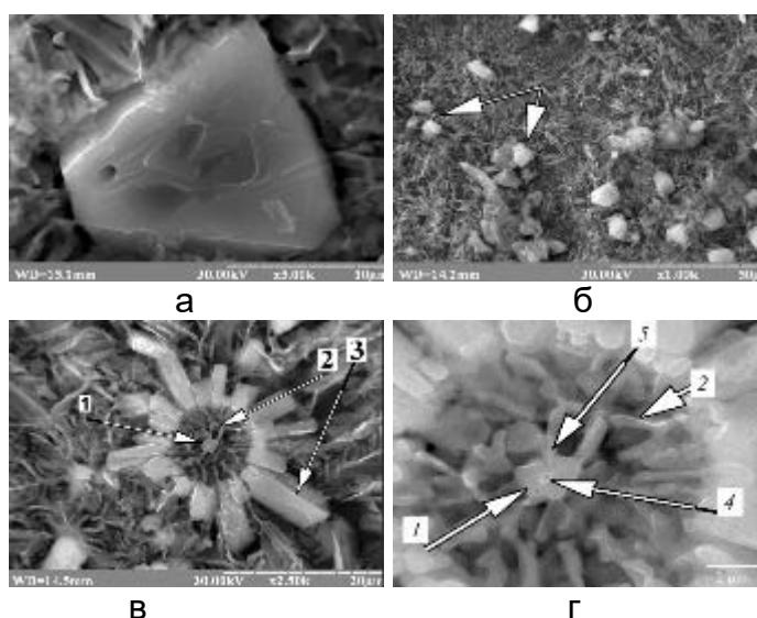
Рис. 4 - СЕМ структура сплаву Al–16,5% Si після деформаційного швидкісного охолодження (електролітичне травлення): а – h = 1 mm; б–д – 0,3 mm.
