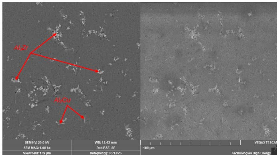
Рис. 2 – Електронно-мікроскопічне зображення мікроструктури сплаву \text{Al} - 5\% \text{Cu} - 0,8\% \text{Mn} - 0,25\% \text{Ti} зміцненого цирконієм із \text{ZrF}_4 (1,8 %)
