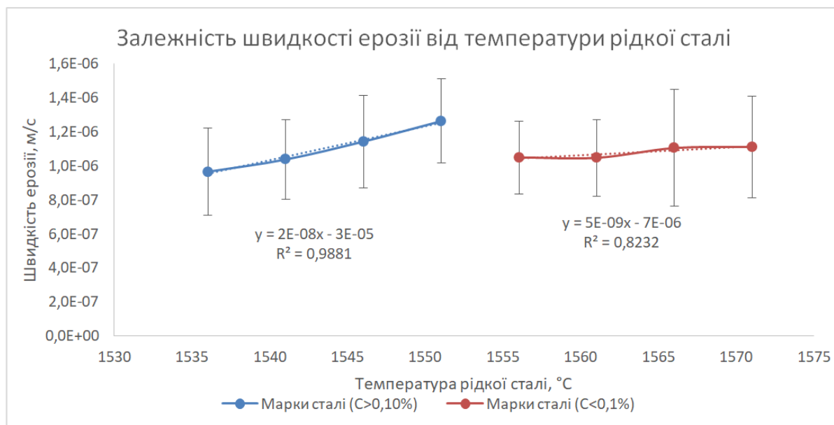
Рисунок 2 – Залежність швидкості ерозії від температури рідкої сталі
