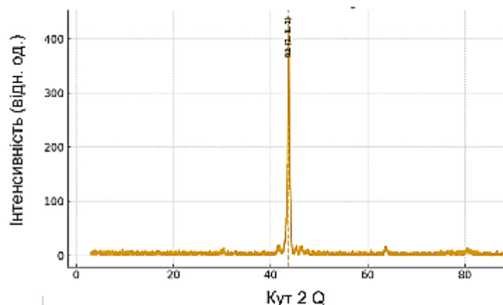
Рис. 1 – Дифрактограма сплаву 1
