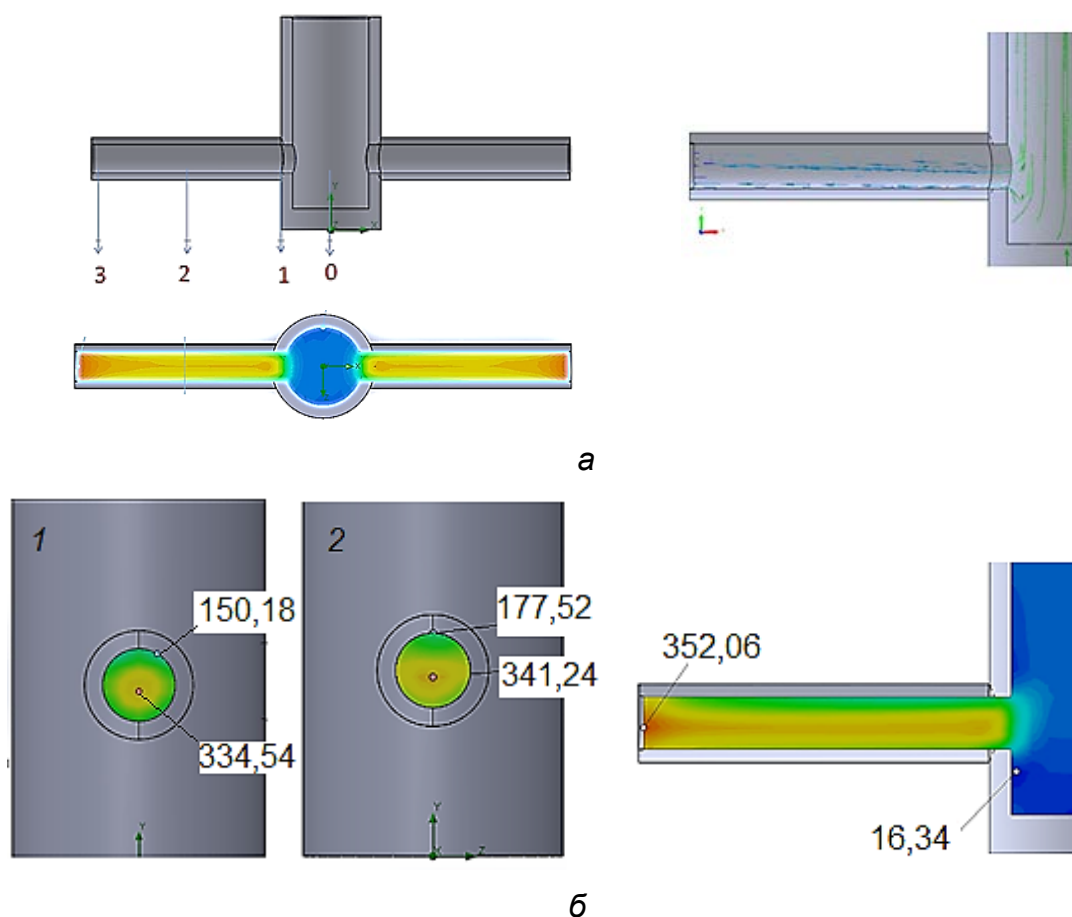
Рисунок 1 – Напрямки (а) та розподіл швидкостей (б) потоку в Т-подібному наконечнику заглибної фурми при тиску газу-носія 0,6 МПа
