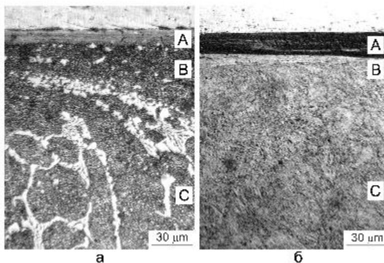
Рис. 1 – Структура зони контактної взаємодії сталей 130X17 (а) і 20X13 (б) після випробувань на тертя. Торцевий шліф. А — зносостійкі самоорганізовані покриття, В — деформований вихідний метал, С — недеформований вихідний метал.
