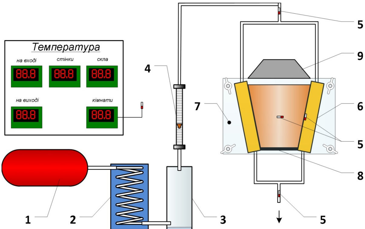
Рисунок 1 – Схема експериментальної установки: 1 – компресор потужністю 1,5 кВт та продуктивністю 200 л/хв.; 2 – охолоджувач повітря; 3 – конденсатор для збирання вологи; 4 – поплавковий ротаметр типу РМ-2,5 ГУЗ; 5 – сенсори електронних термометрів; 6 – мідні холодильники; 7 – скляні пластини; 8 – гумове днище; 9 – абажур з лампою на 12 Вт для підігріву верхньої частини зразка
