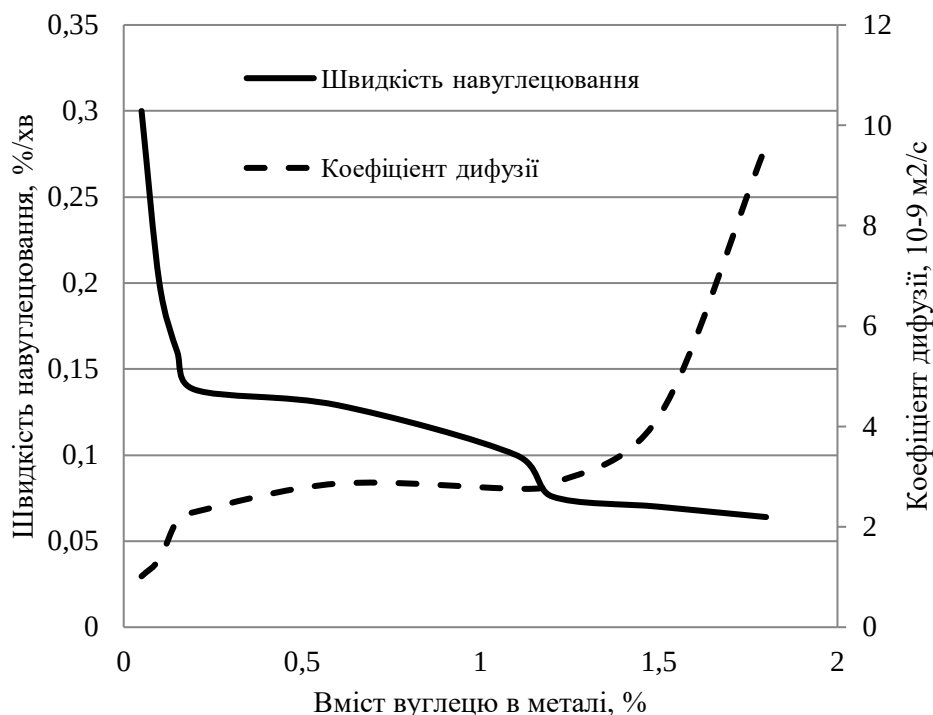
Рисунок 1 – Залежність швидкості науглецювання металу і ефективного коефіцієнту дифузії від вмісту вуглецю в металі.
