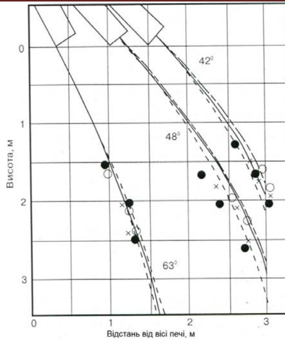
Рис. 1 – Порівняння результатів розрахунків та вимірювань на фізичній моделі БЗП: — — — , ● - кокс; — — — , х — агломерат; — ■ —, О - окатиші. Цифри у кривих – кут нахилу лотка, град.
