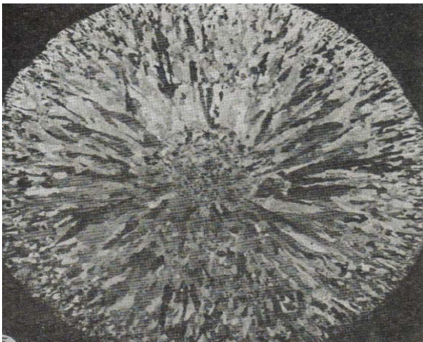
Рис.1. Макроструктура зливку хромового сплаву ВХ-2И, виплавленого в дуговій печі з витрачаємим електродом, в атмосфері аргону.
