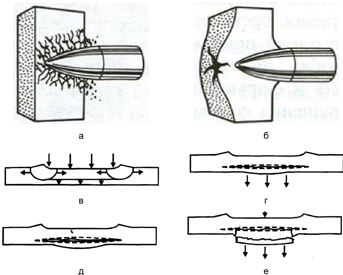
Рис. 1. Види руйнування відколом (а, б) і етапи утворення та відриву
