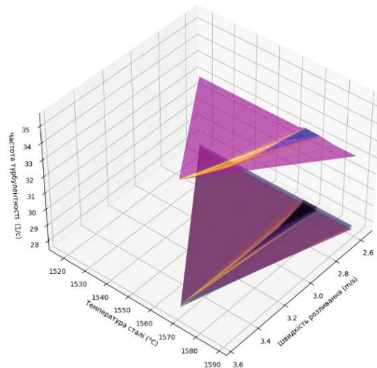
Рисунок 5 Залежність частоти турбулентної енергії від температури та швидкості розливання
