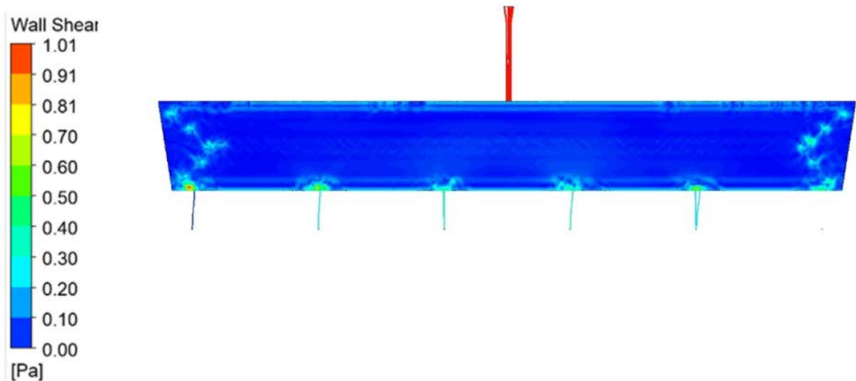
Рисунок 2 – Розраховане напруження зсуву зони випускних отворів проміжного ковша
