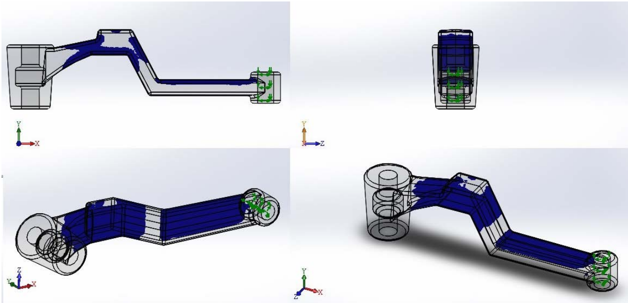
Рис.1 – Розподіл навантаження в об'ємі виливка
