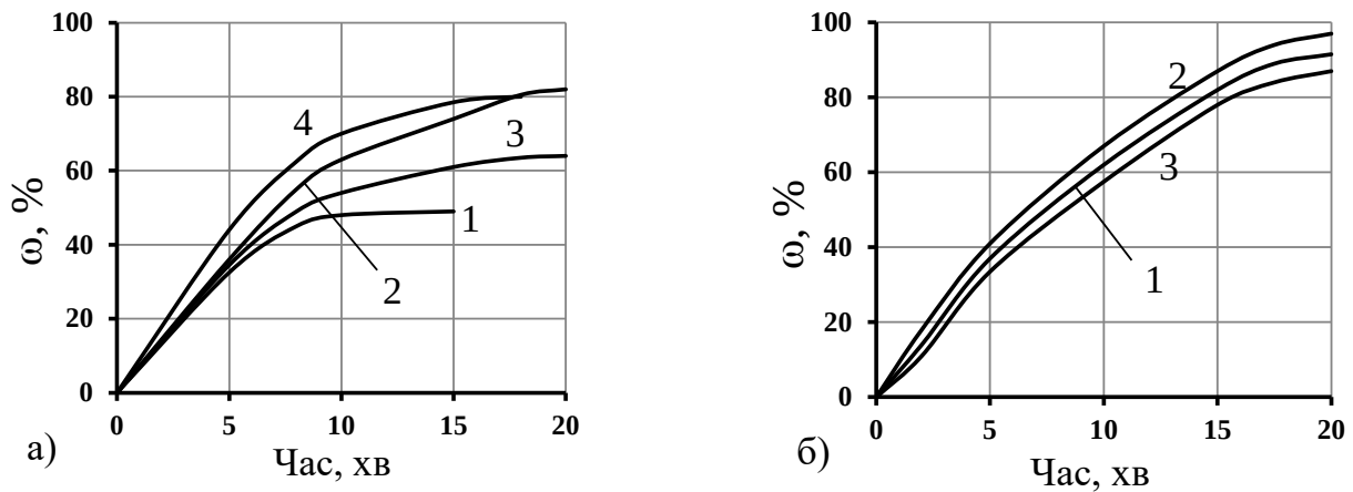
Рисунок 1. Кінетика окислення заліза, отриманого в різних умовах, при температурах, що відповідають T_{ок} : а) отримано відновленням магнетитового концентрату воднем: 1,2 – 773 К, 3,4 – 873 К, 1,3 – без добавки, 2,4 – 1 % KCl; б) залізо отримано відновленням Fe_3O_4 воднем при 873 К: 1 – без добавки, 2 – 1 % KCl, 3 – 1 % LiCl
