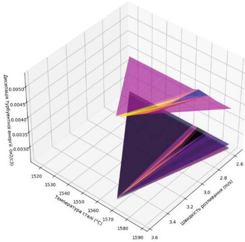
Залежність дисипації турбулентної енергії від температури та швидкості розливання (Зони 1-4)
