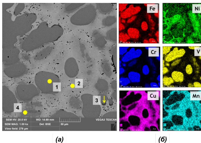
Рис. 2 – Фотографія СЕМ мікроструктури (а) та кольорові карти розподілу елементів (б) литого високоентропійного сплаву \text{Fe}_{18}\text{Ni}_{18}\text{Cr}_{18}\text{Cu}_{18}\text{Mn}_{18}\text{V}_{10} .
