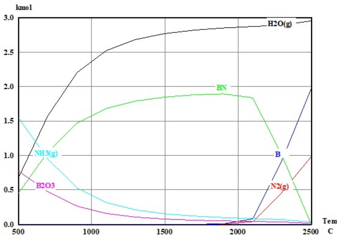
Рисунок – Рівноважний склад системи B-O-H-N при синтезі нітриду бору з використанням карбаміду.
