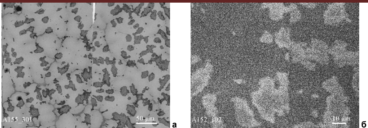
Рис.2. Структура зразків, отриманих зварюванням кубиків багатокомпонентного сплаву системи Nb-Cr-Ti-Al-Mo ( T_{д.з.} - 1200^{\circ}\text{C} , P_{д.з.} - 125 \text{ МПа} , t_{зв.} - 30 \text{ хв.} , вакуум - 4 \cdot 10^{-3} \text{ Па} ): а - BEI; б - X-ray Ti-K _{\alpha}
