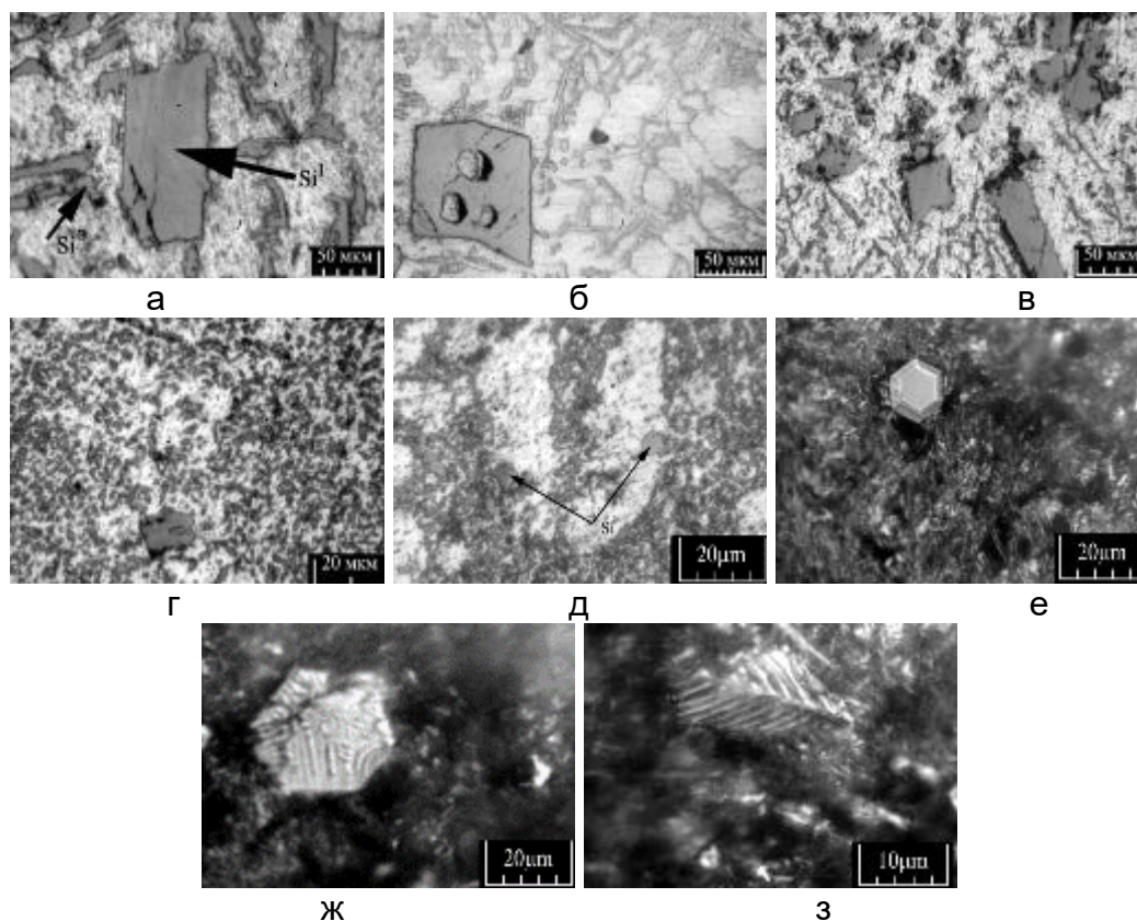
Рис. 2 – Мікроструктури сплаву Al–16,5 % Si після традиційного охолодження (а, б) та деформаційного швидкісного охолодження (в–з) за різної локальної товщини зразка h : а, б – традиційне охолодження; в – 1 мм, г – 0,5 мм, д–з – 0,3 мм; а–е – хімічне, е–з – електролітичне травлення.
