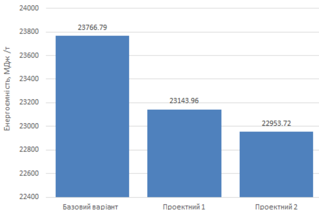
Рисунок 1 – Енергоємність сталі марки 5ПС для умов ПрАТ «ДМЗ»
