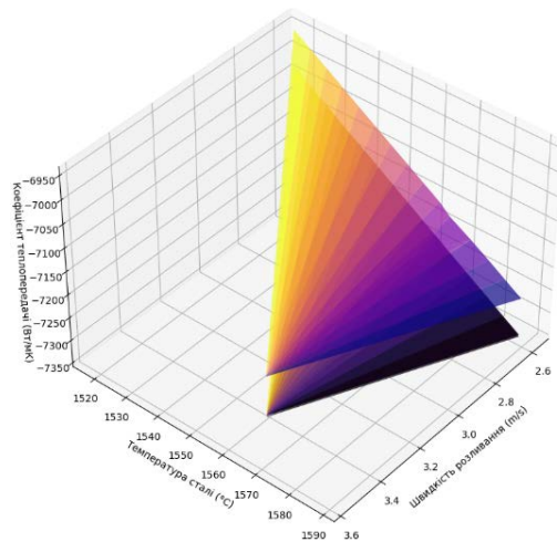
Рисунок 6 Залежність коефіцієнта теплопередачі від температури та швидкості розливання
