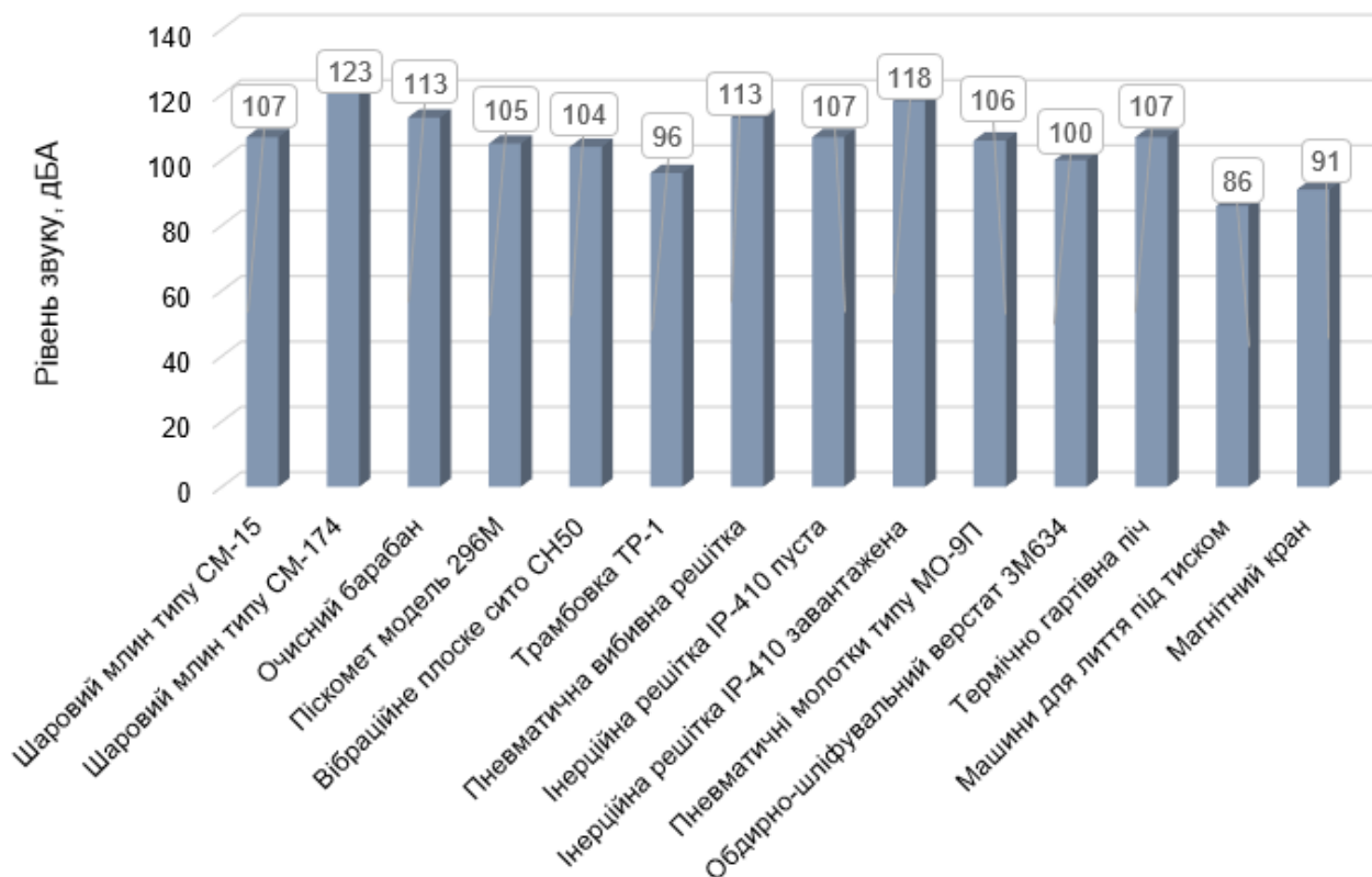
Рис.1 – Рівень звуку для різних видів виробничого обладнання у приміщеннях ливарних цехів
