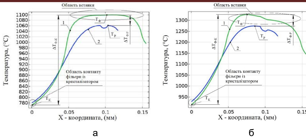
Рис. 1 – Графіки залежності зміни температури фільєри в залежності від відстані вздовж осі ОХ при часі нагріву ( \tau ) 2000 с: а – з використанням сталюї вставки, P = 6,6 кВт); б – з використанням графітової вставки, P = 12,3 кВт. (1 – на поверхні фільєри; 2 – на нижній поверхні фільєри, яка контактує з розплавом)
