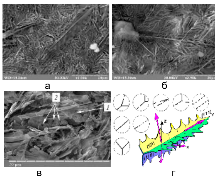
Рис. 3 - СЕМ структура сплаву Al–16,5% Si після деформаційного швидкісного охолодження ( h = 0,3 mm): а – дві видимі площини кремнієвого дендриту;
