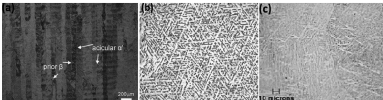
Рис. 1 – Мікроструктура зразків Ti-6Al-4V у стані «as-built» після SLM, EBM та DED [7].
