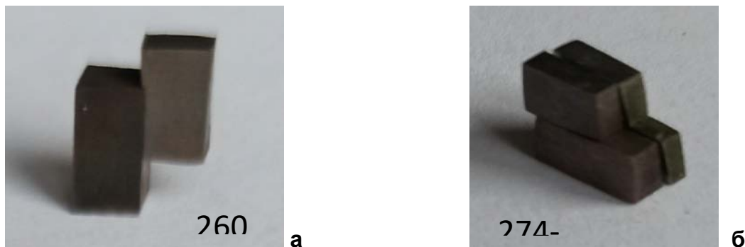
Рисунок 1 – Зразки для дослідження дифузійної зони і впливу її структури на міцність з'єднання: а – зразок після дифузійного зварювання; б – після розрізання на половинки
