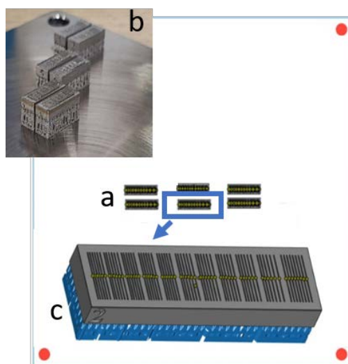
Рисунок 1 - Схема розташування поодиноких треків з різними режимами (а), загальний вигляд ділянки зі зразками в робочій камері (b) та зовнішній вигляд дослідних зразків (с)
