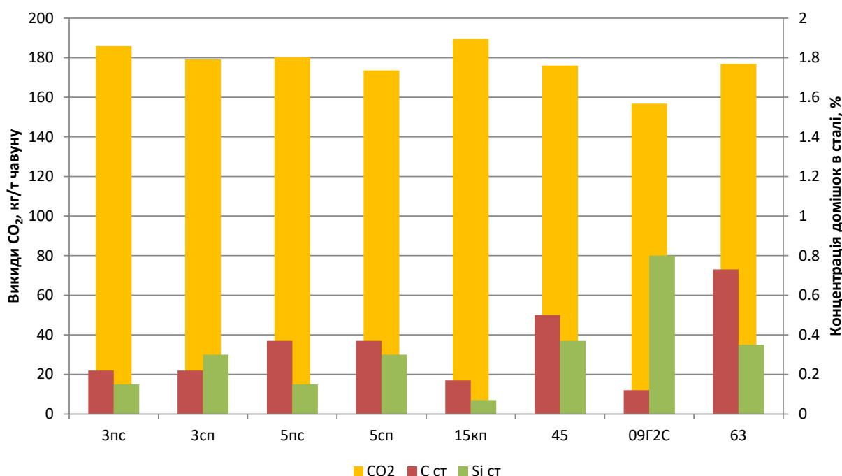
Рисунок - Питомі викиди \text{CO}_2 при отриманні сталі в КК
