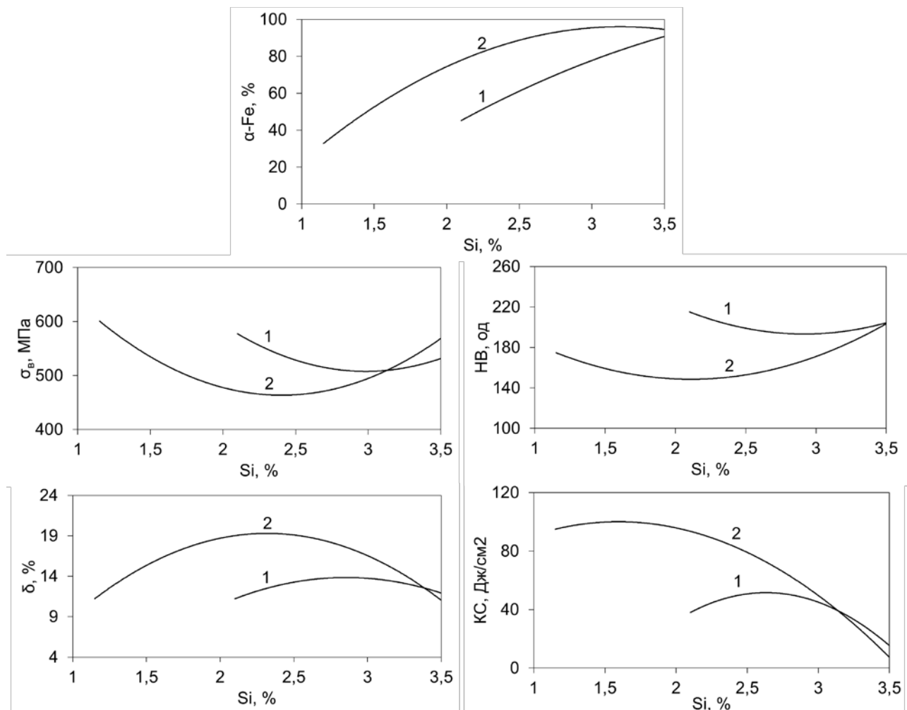
Рис. 1 – Вплив масової частки Si на структуру та механічні властивості високоміцного чавуну в клиноподібних пробах товщиною 25 мм при методах модифікування у ковші (1) або в ливарній формі (2)
